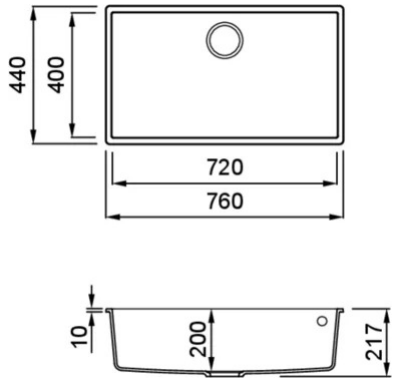
Disegno tecnico
