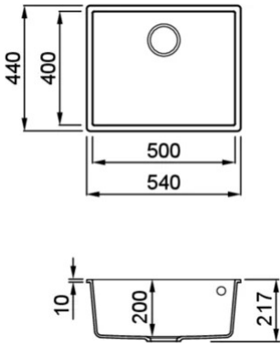
Disegno tecnico
